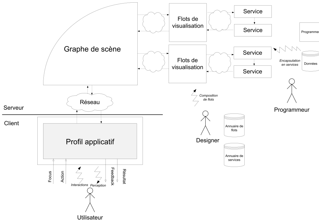
FIGURE 5.1 – Aperçu de l'architecture VizOD.
