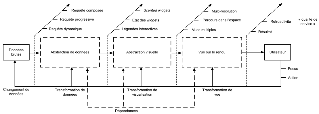
FIGURE 3.14 – Synthèse de l'espace d'interaction visuelle.
