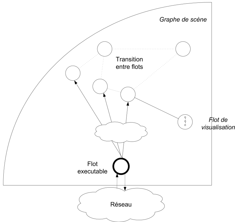
FIGURE 5.5 – Schéma d'un graphe de scène.
