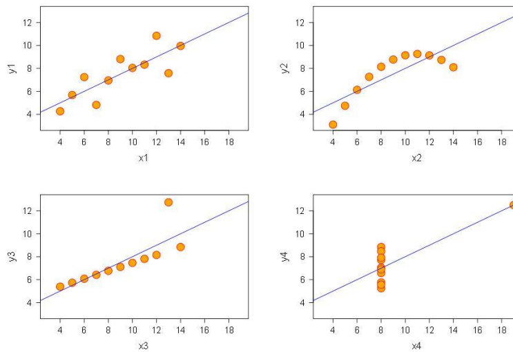
FIGURE 4.4 – Représentation graphique du Anscombe's Quartet .
